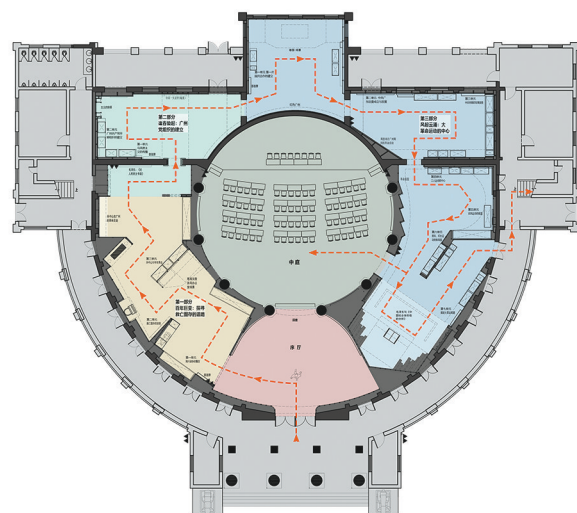
展厅一层平面图
